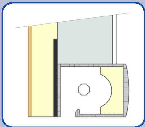
Principe du coffre de bloc-baie, isolation par l'extérieur
