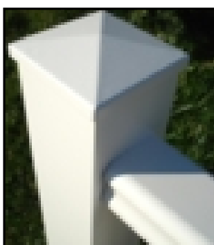
Détail tête de poteaux + lisse haute 71x52 mm
